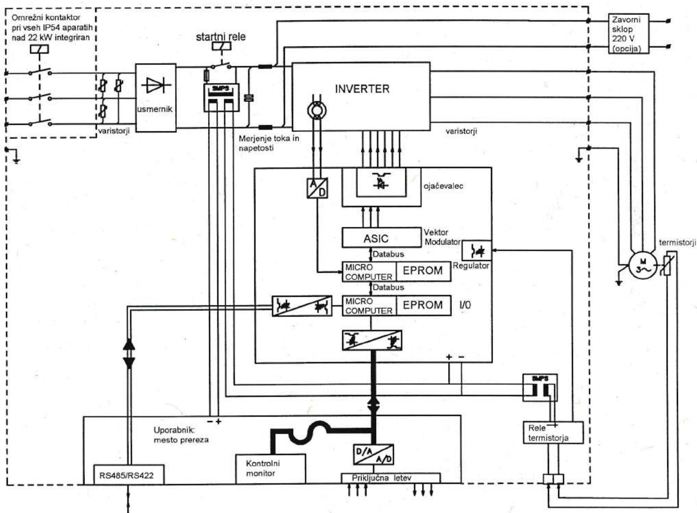
Slika 14.8 Funkcijski diagram
